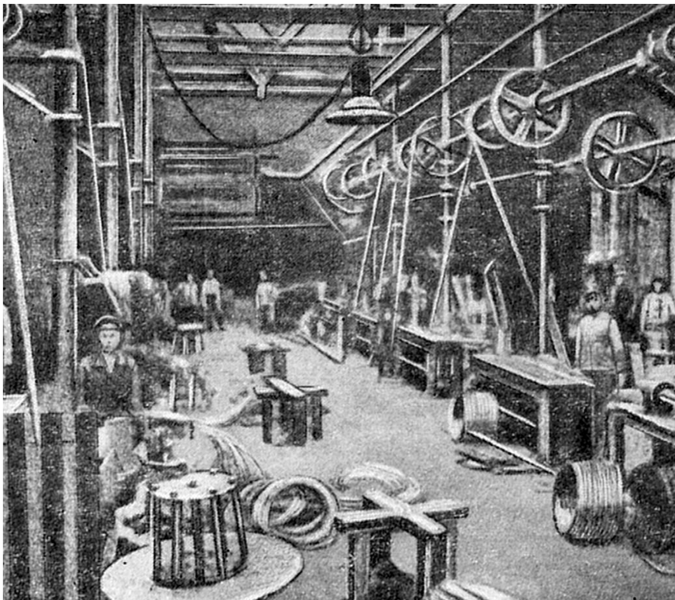
Волоочильный цех завода Электропровод
